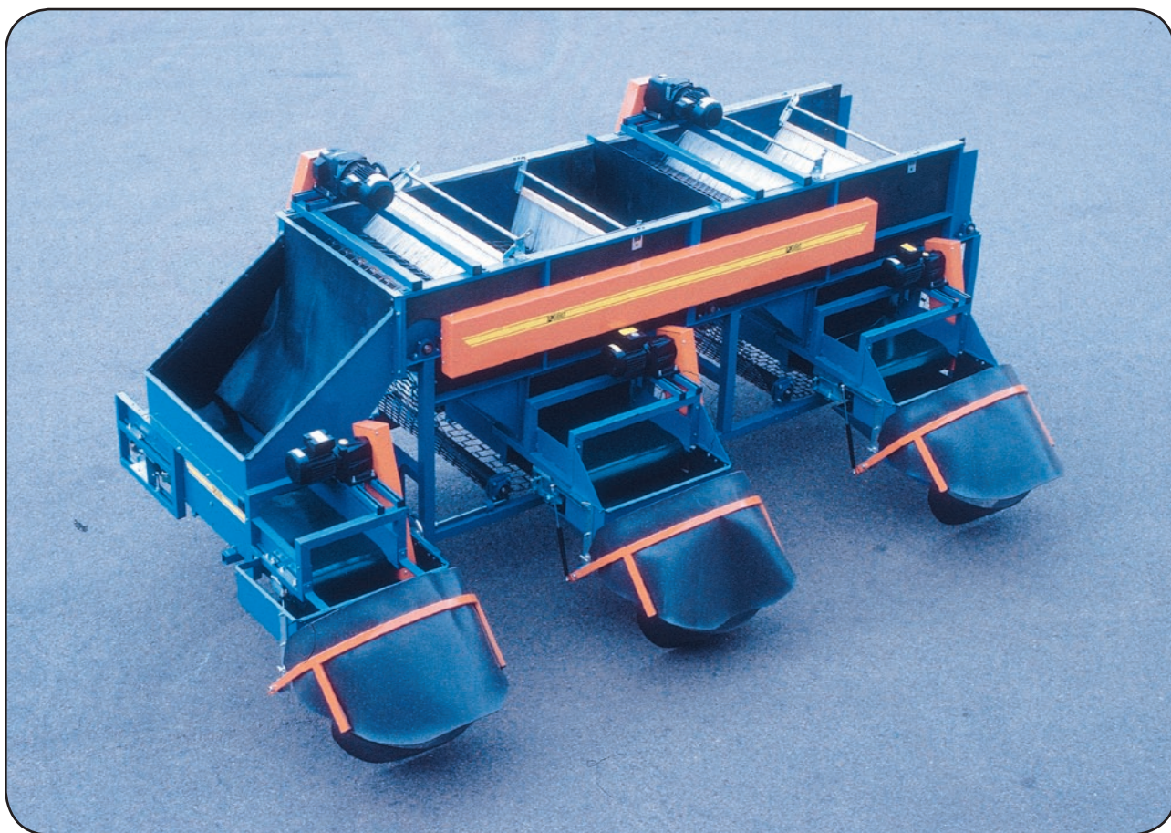
Nätsorterare G B800x2 försedd med transportörer, trattar och falldämpare.
